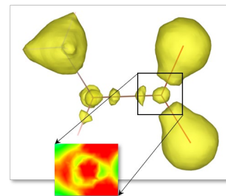
図3 観測されたグリシン分子の価電子密度分布
