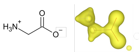
図2 睡眠の質を高めるアミノ酸：グリシン 左は化学構造式、右はソフトウェアVESTAで描いた電子分布のモデル図
