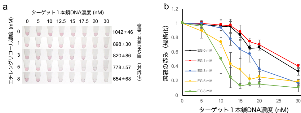
図 異なる修飾 DNA 量の金ナノ粒子によるターゲット 1 本鎖 DNA 検出. a) エチレングリコールにより修飾 DNA 量を制御した金ナノ粒子に対して、様々な濃度のターゲット 1 本鎖 DNA を加えたときの溶液色変化. b) a)の溶液色画像を色分解し、赤青緑成分強度より求めた赤み (=赤-(緑+青)/2)
