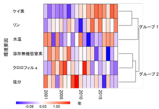
補足図2. 燧灘の環境要因に関する経年変化(2001~2019年5~7月)。 クラスター分析から、環境要因は2つのグループに分けられ、最近年(2010年以降)では溶存無機態窒素が減少すると同時に、クロロフィルa(植物プランクトン)も減っていることが判りました(低: 青→白→赤: 高)。
