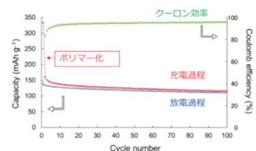
図2 分子1を正極活物質とする二次電池のサイクル特性
