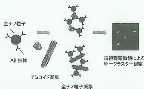
図 金ナノ粒子凝集を利用した、単一クラスター観察によるタンパク質アミロイド凝集の高感度検出
