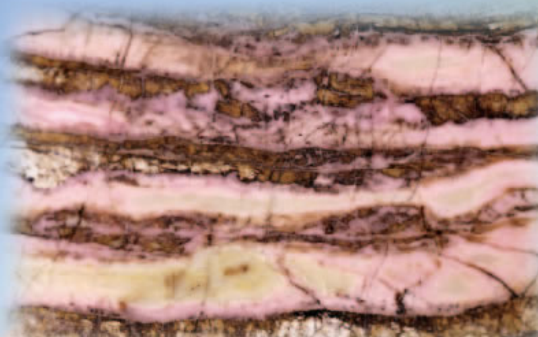
バラ輝石
