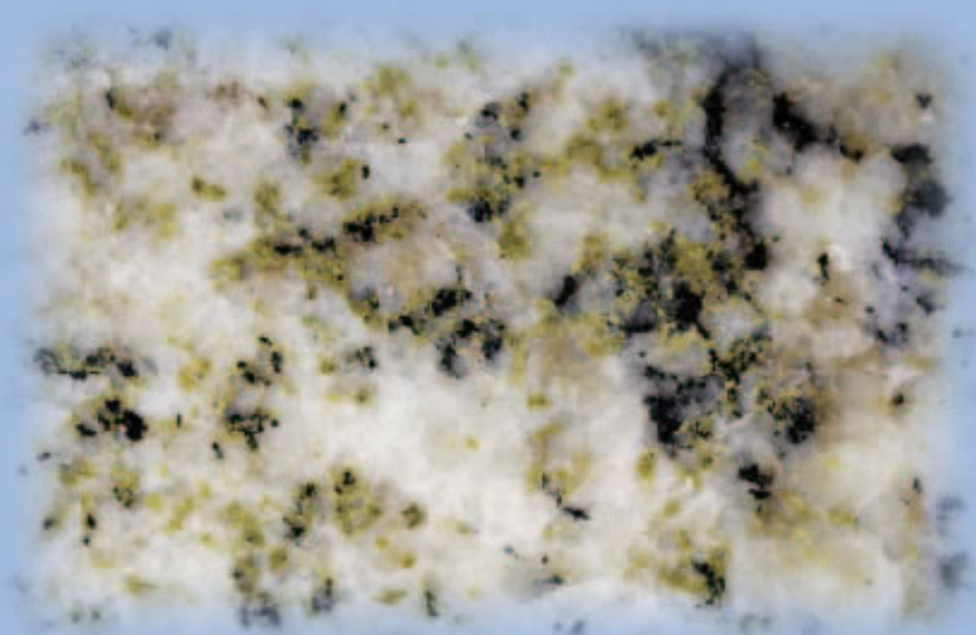
杉石
