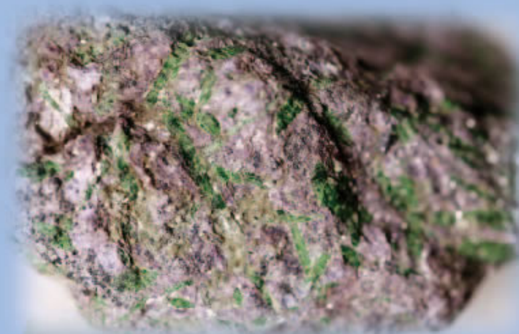
愛媛閃石
