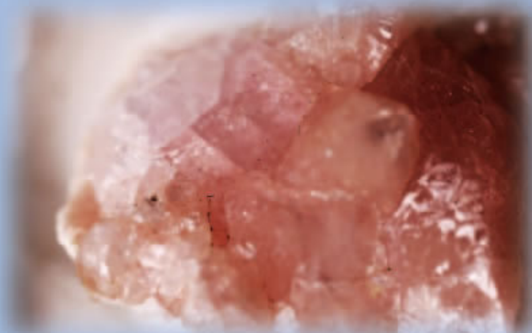
魚眼石
